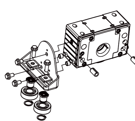
DRS112-200 Horizontal Guide Rollers
